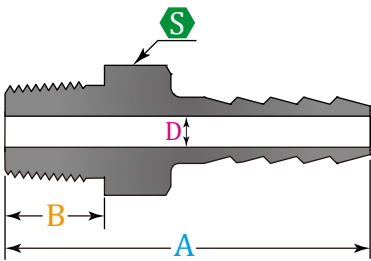
锥螺纹终端橡胶管接头
