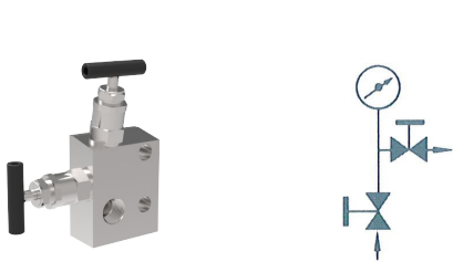
二阀组 EF-3
