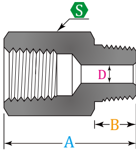
内外接头（二）
