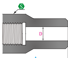
双金属温度计管嘴
