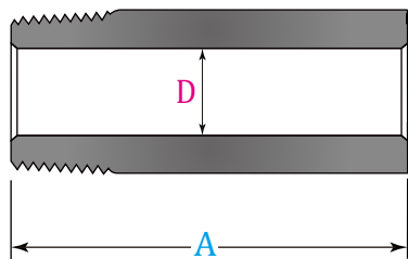
单头异径短节
